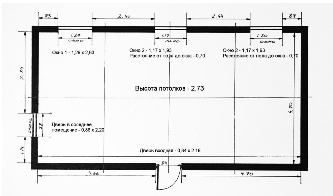
Чертеж помещения 2
