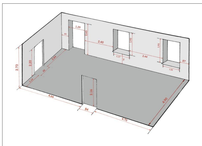
Чертеж помещения 2
